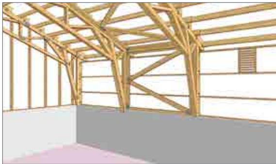
Bilde: Viser avstivning av vegg og tak.
