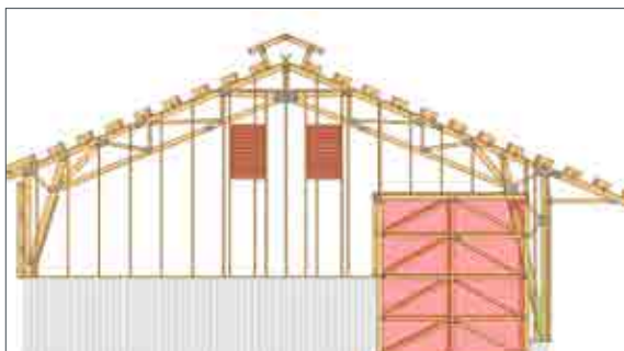
Bilde: Viser galvvegg med port.
